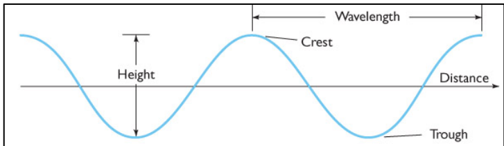
(a) WAVE PARAMETERS
